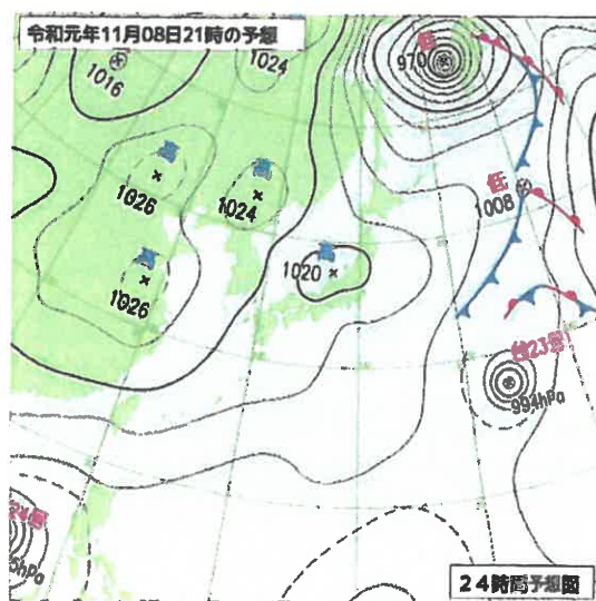
予想天気図（8日21時）
