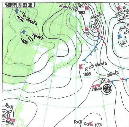
実況天気図（8日3時）
