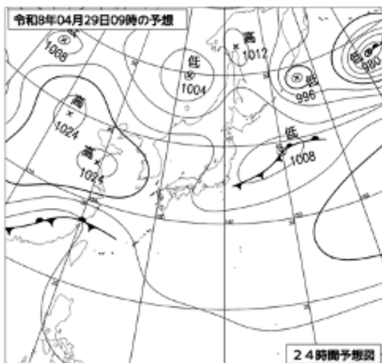
4月29日 09時 の予想天気図
